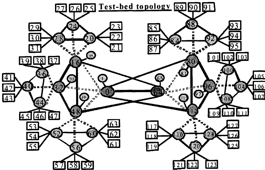
Figura 5.1: Topologia utilizada no Exemplo 1
